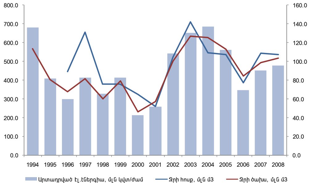
Գծանկար 1. Սարսանգ ՀԷԿ-ի հիմնական ցուցանիշները
